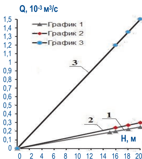
Рисунок 5 – Графики Q = f(H) :
